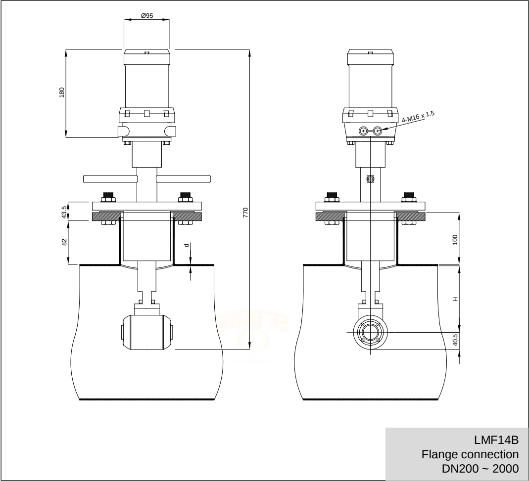
LMF14B - Dimension (mm)
