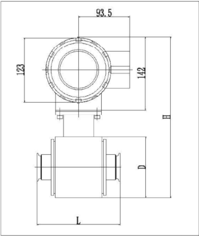
LMF13 - Dimension (mm)
